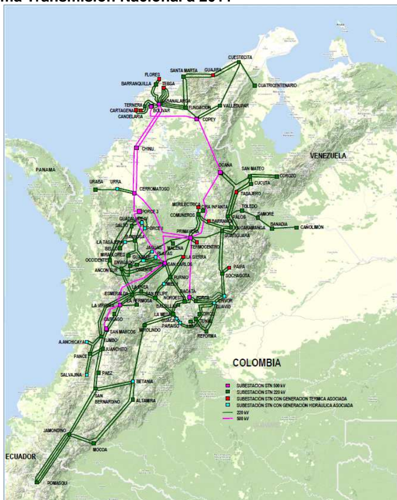
Figura 1 Sistema Transmisión Nacional a 2011
